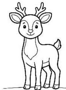
Deer Venado
